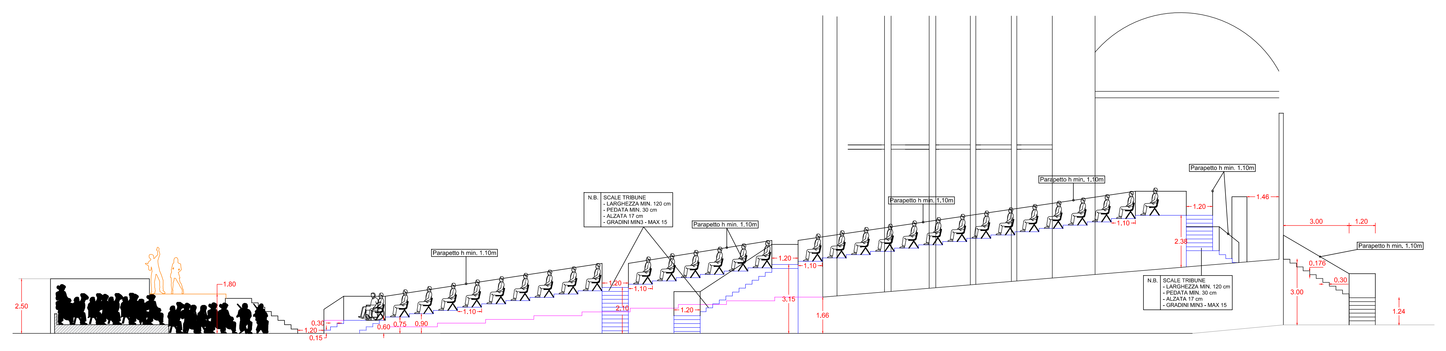
SEZIONE TRIBUNA 1:100
