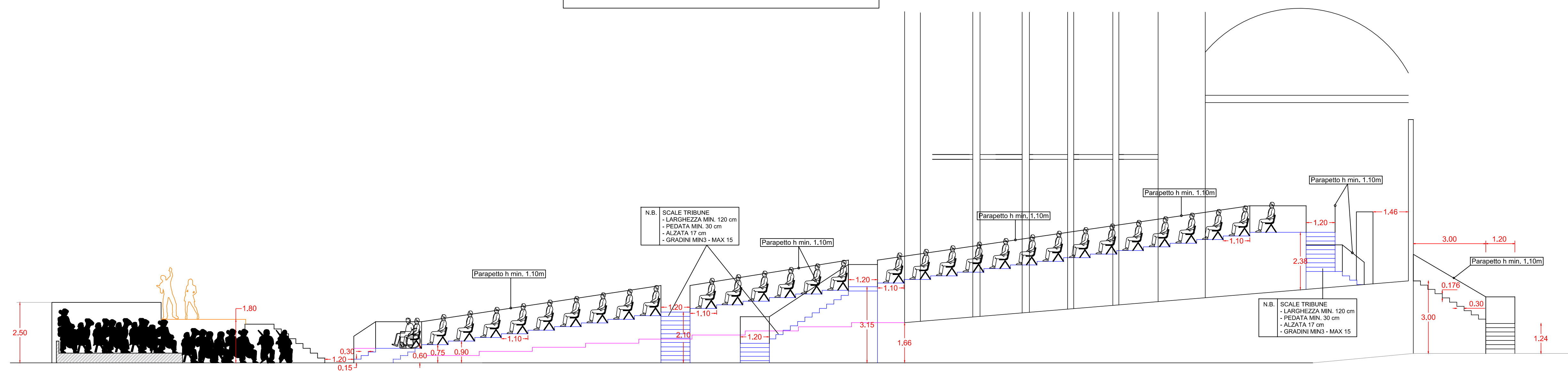
SEZIONE TRIBUNA 1:100
