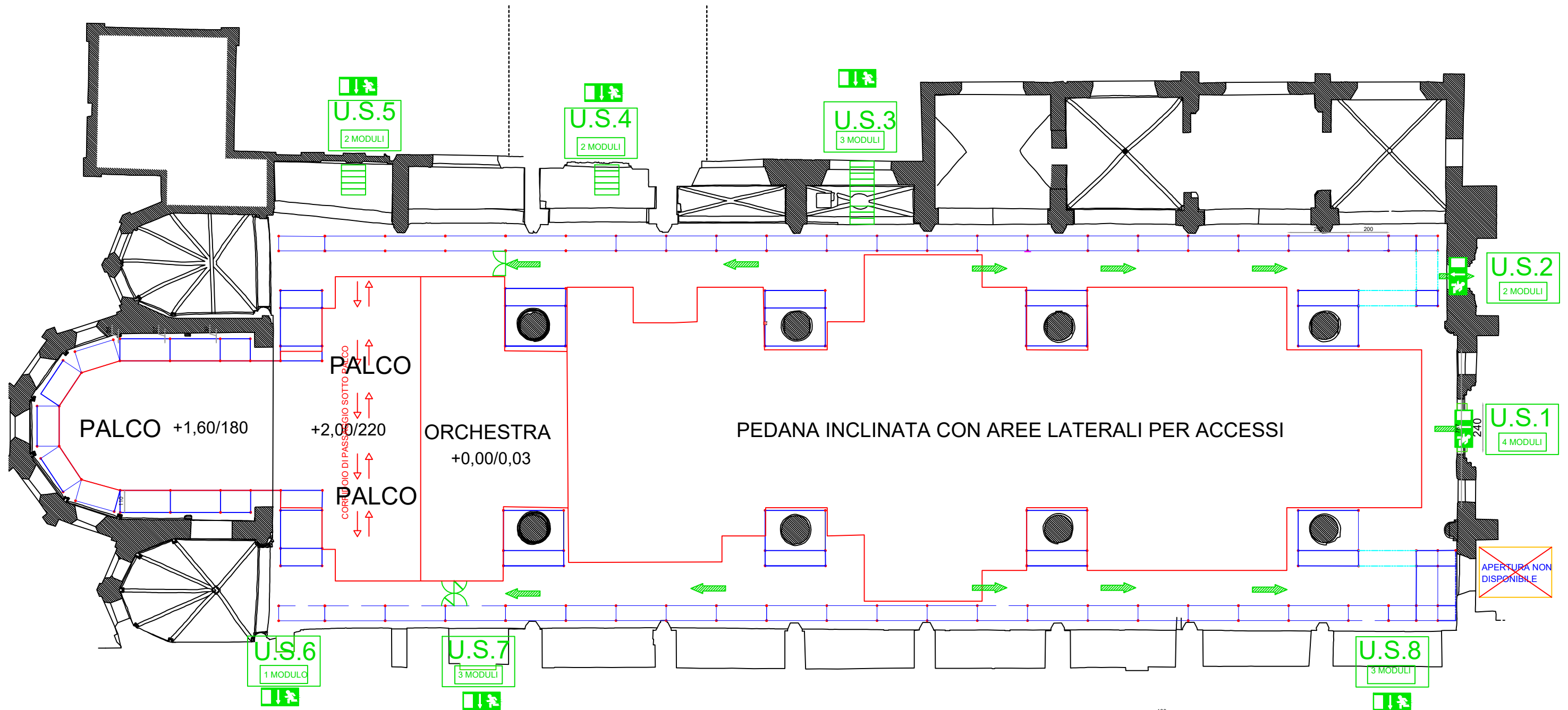
PIANTA 1 LIVELLO
